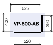
VP-600 High lid AB. BUSCH pump 20m³/h.
