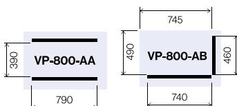
VP-800 High lid AB, AA. BUSCH pump 63m³/h.
